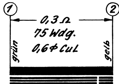
Siebdrossel BV 48/28
