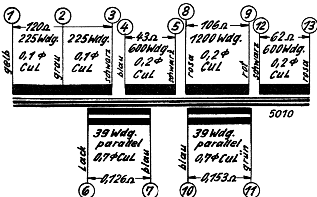
Tiefen-Übertrager BV 78/44
