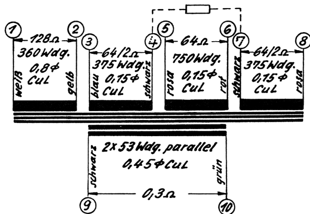
Mittelfrequenz-Übertrager BV 48/35
